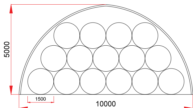
15 x Ø1.50 m
