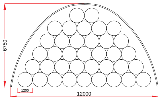
37 x Ø1.20 m
