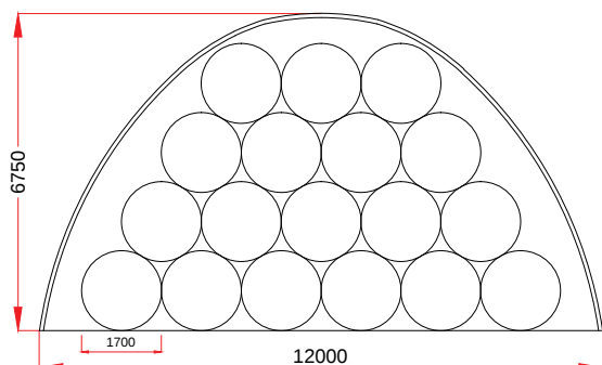
18 x Ø1.70 m
