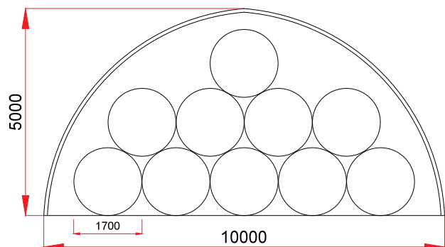
10 x Ø1.70 m
