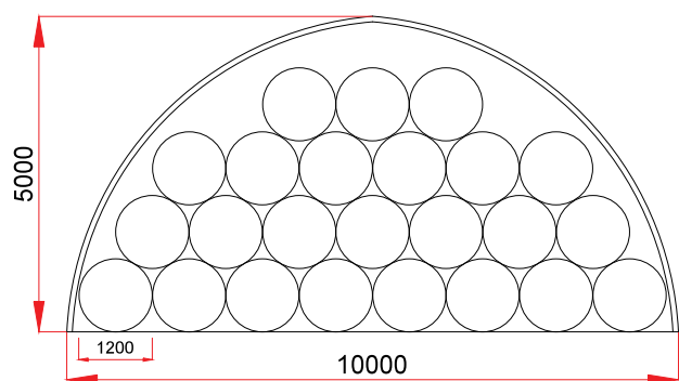
24 x Ø1.20 m
