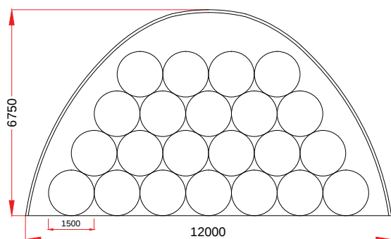
22 x Ø1.50 m
